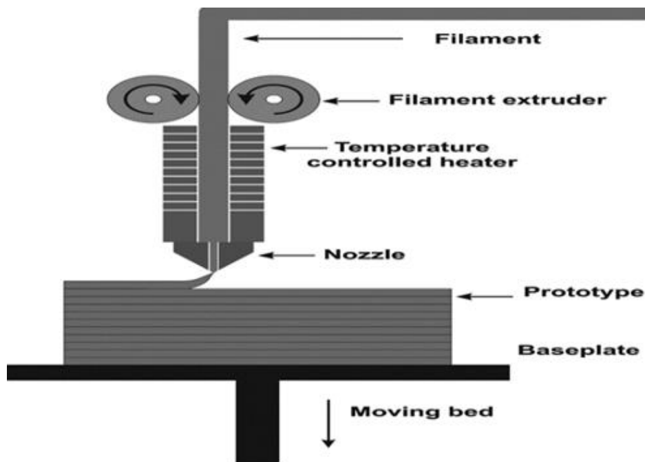
Figura III: Esquema de impressão 3D pelo método FDM
